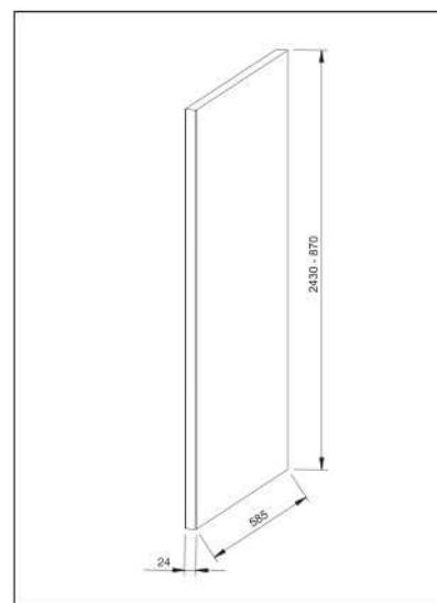
Završni panel
