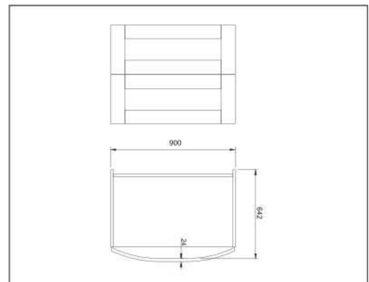
Zaobljeni par dubokih ladica
