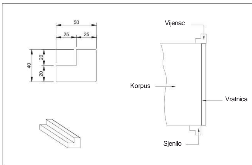
Vijenac i sjenilo
