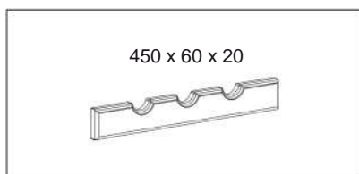
Držac boca
