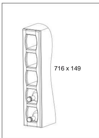
Okvir držača za boce
