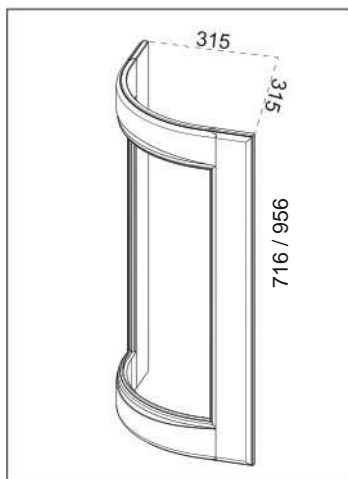
Zaobljeni par okvira
